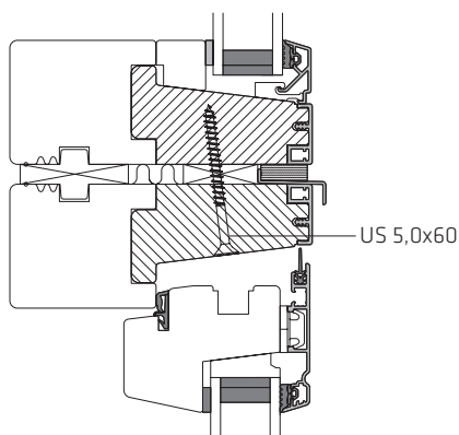
VANDRET SAMLING, MED LISTE
