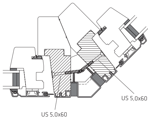
45° HJØRNELØSNING
