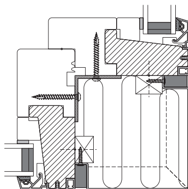
90° HJØRNELØSNING
