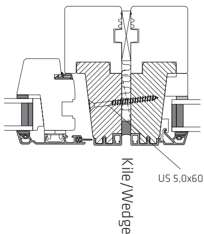
LODRET SAMLING, MED LISTE OG FUGE
