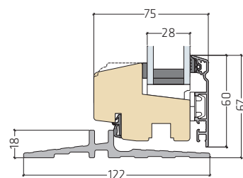
FRAic20-13L28 | Lavt bundtrin terrassedør
