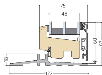
FRAic20-13L48 | Lavt bundtrin terrassedør
