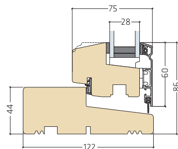
FRAic20-10L28 | Bundtrin terrassedør
