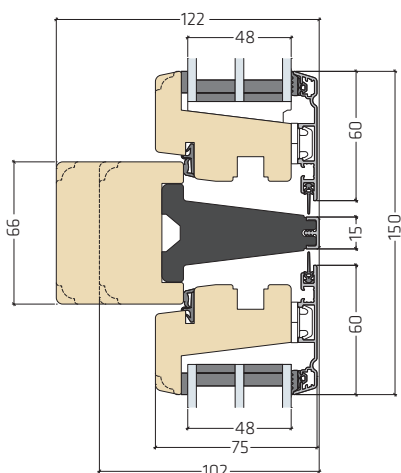
FRAic01-40L48 | Vandret post
